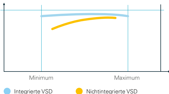
Kombinierte Effizienz Motor/Umrichter
