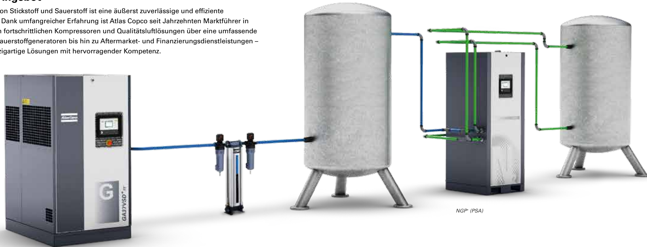
Typische Installation: Kompressor mit integriertem Trockner, Vorfilter UD+, Aktivkohleabsorber QDT, Staubfilter, Behälter, NGP*-Stickstoff-PSA-Generator, Behälter.
